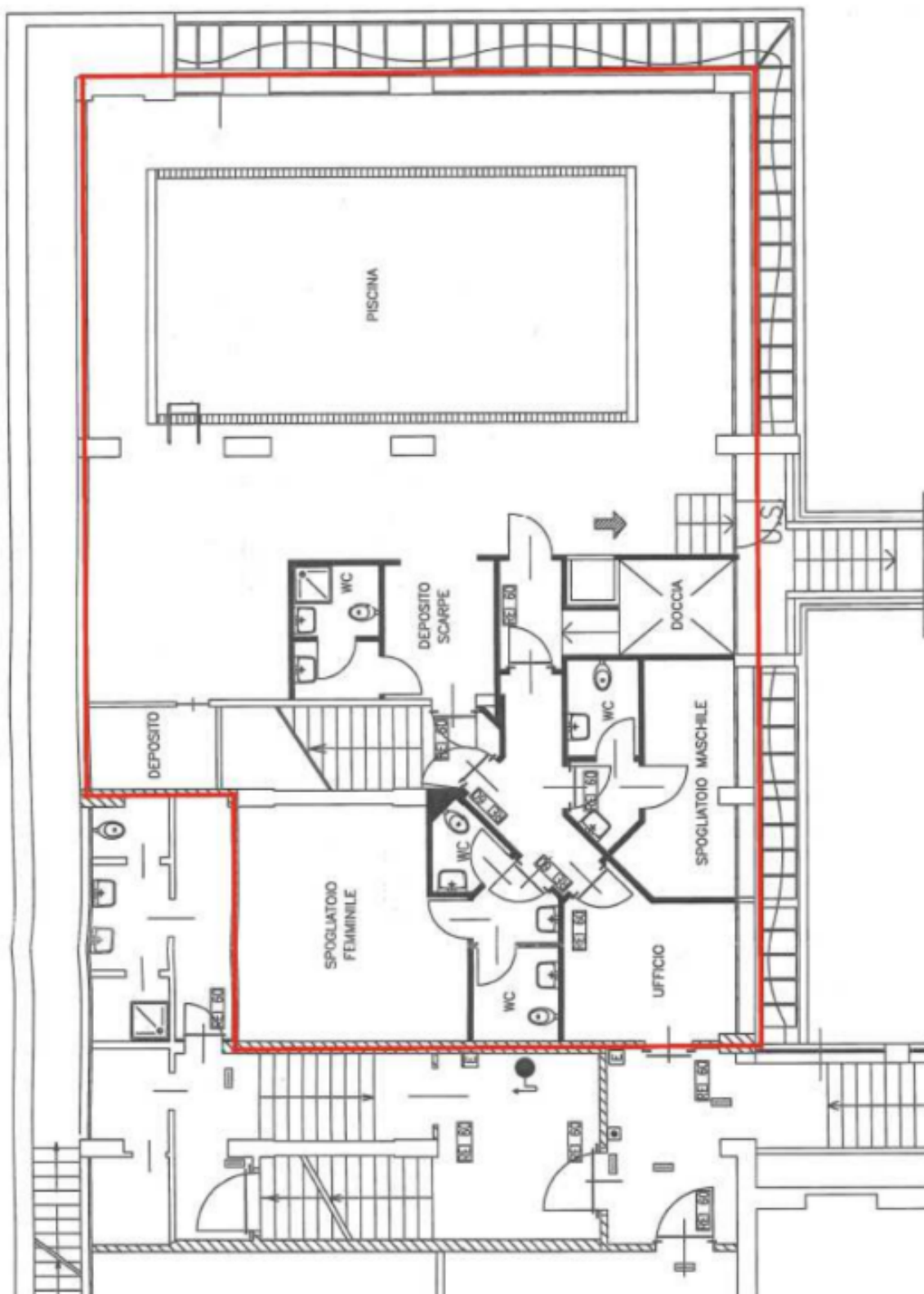
Planimetria
