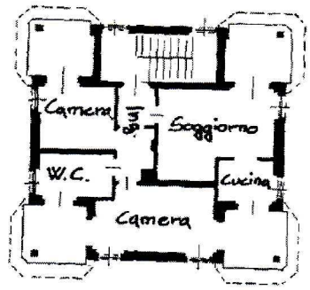
Pianta piano primo h = 2.70
