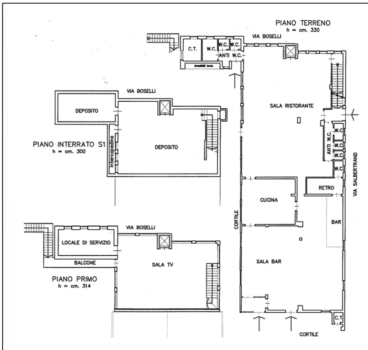
Planimetria indicativa dell'area e dei fabbricati dell'impianto (fuori scala)
