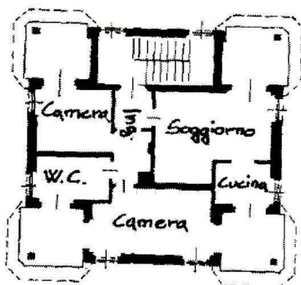
Pianta piano primo h = 2.70
