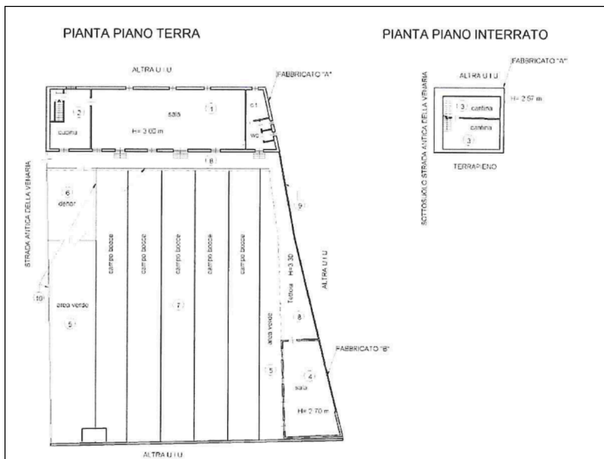
Planimetria generale dell'impianto
