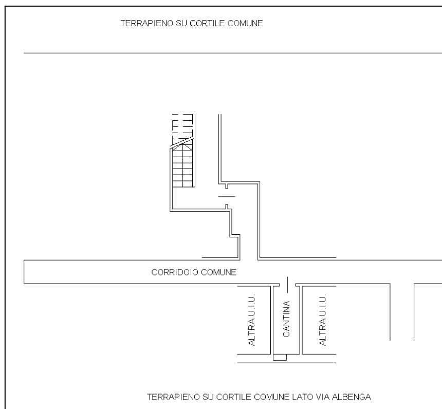
Foglio 1423, particella 236, sub. 399 - Stralcio planimetria C.F. piano interrato - Non in scala
