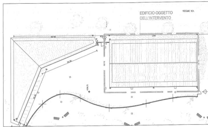
PLANIMETRIA GENERALE - scala 1:200
