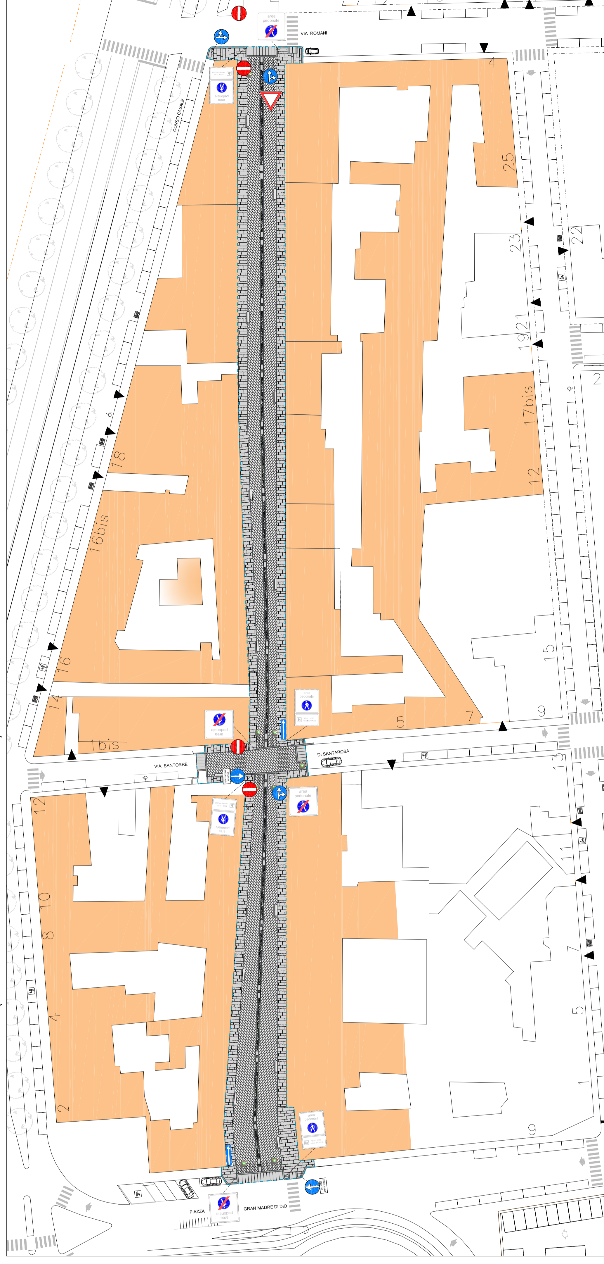
PLANIMETRIA SEGNALETICA VERTICALE (TRATTO PIAZZA GRAN MADRE- VIA ROMANI) - scala 1 : 500
