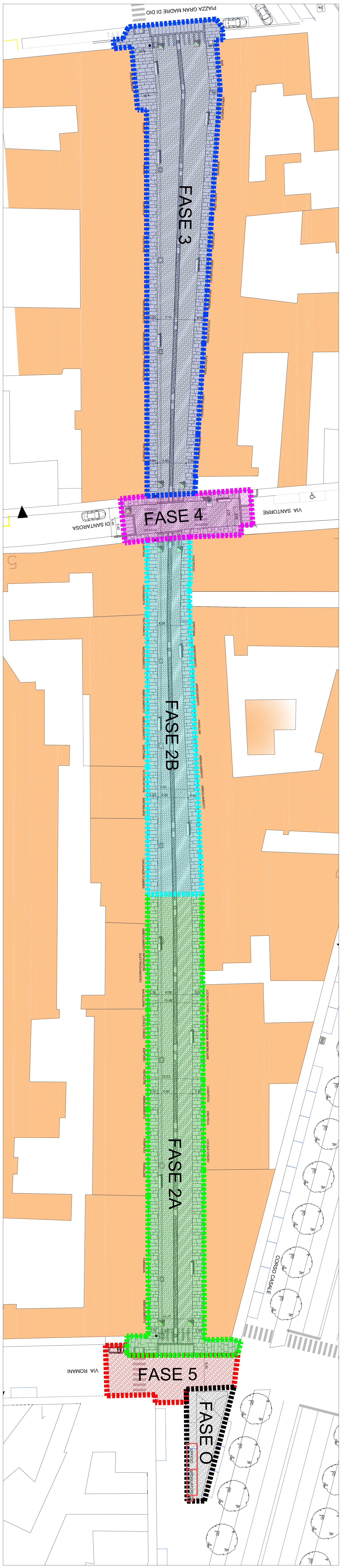
PLANIMETRIA FASI DI CANTIERE TRATTO PIAZZA GRAN MADRE - VIA ROMANI - VIA BRICCA - scala 1 : 200
