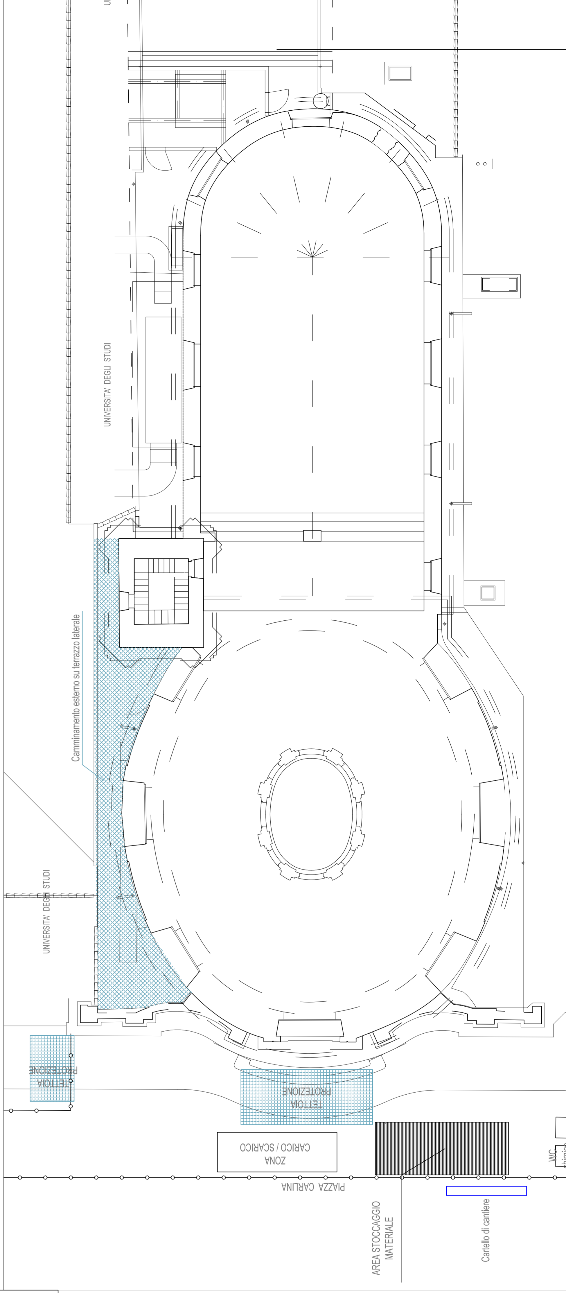
PIANTA PIANO IMPALCATO PONTEGGIO
