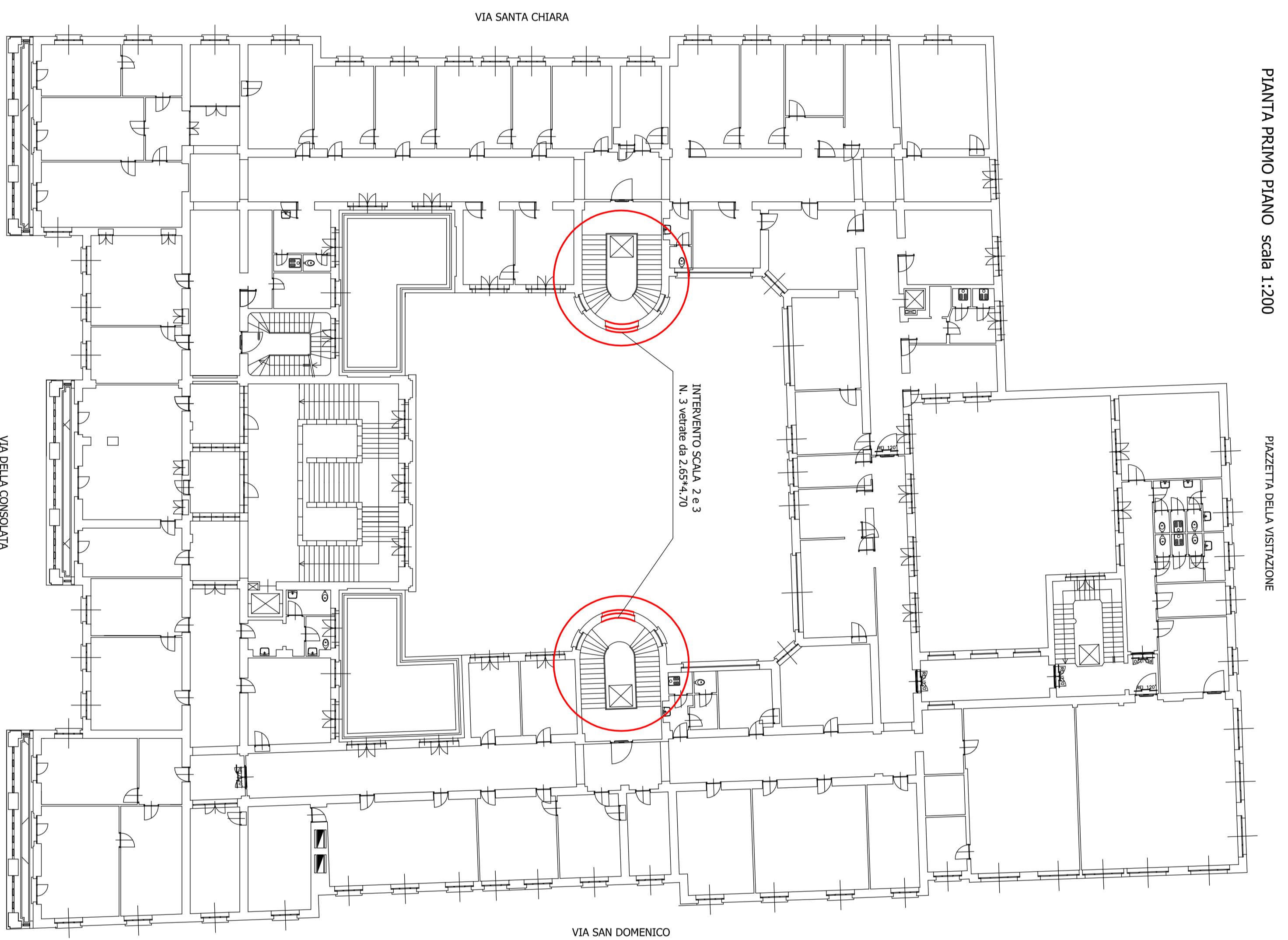
PIANTA SECONDO PIANO scala 1:200
