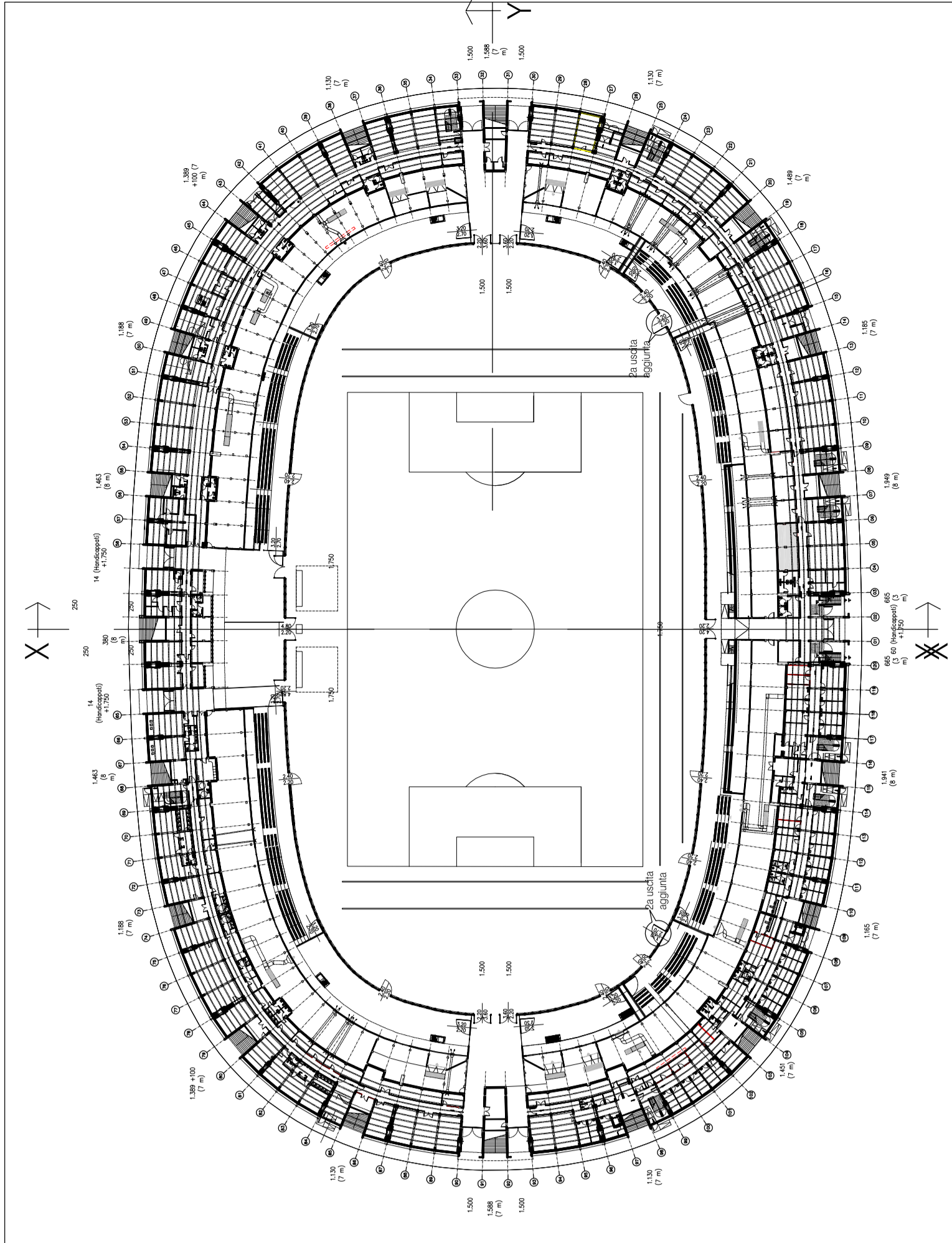
PIANTA COPERTURA - scala 1:1000
