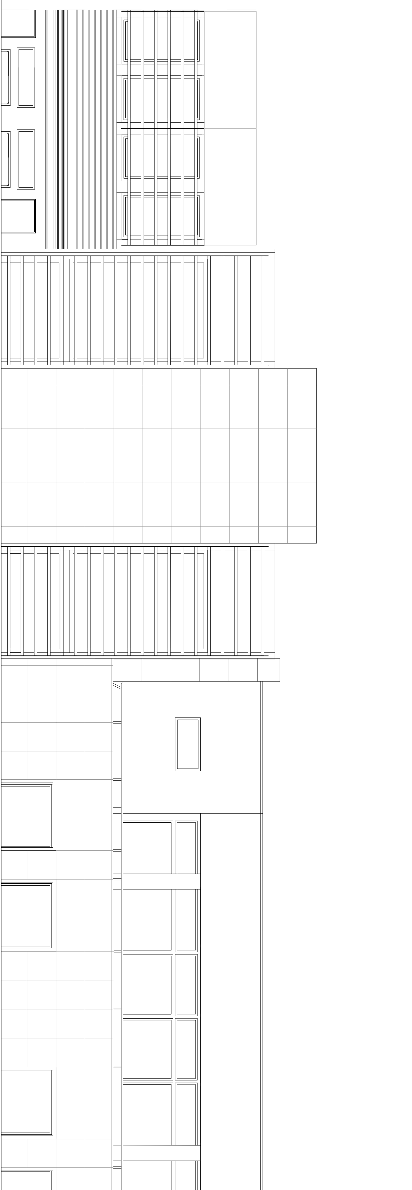
ESTRATTO PROSPETTO SU CORTILE scala 1:50
