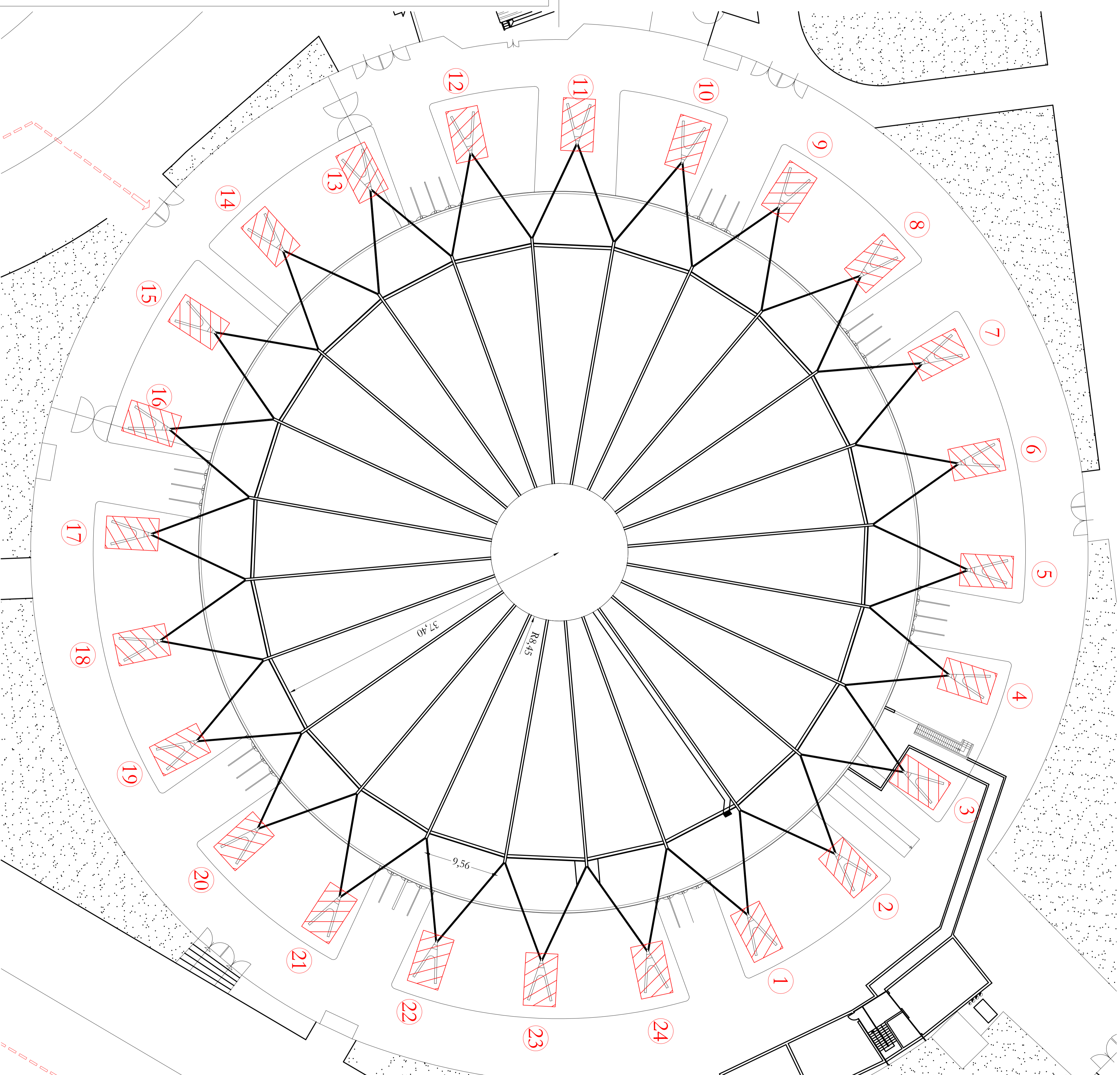
PLANIMETRIA GENERALE 1:250
