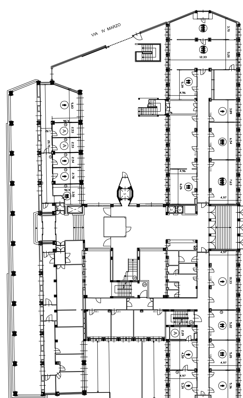
PIANTA PIANO REALZATO - realizzazione di nuovo pavimento vaticco omogeneo completo
