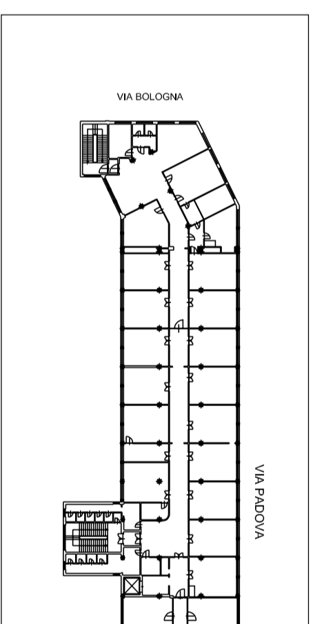
PLANIMETRIA GENERALE PIANO PRIMO
