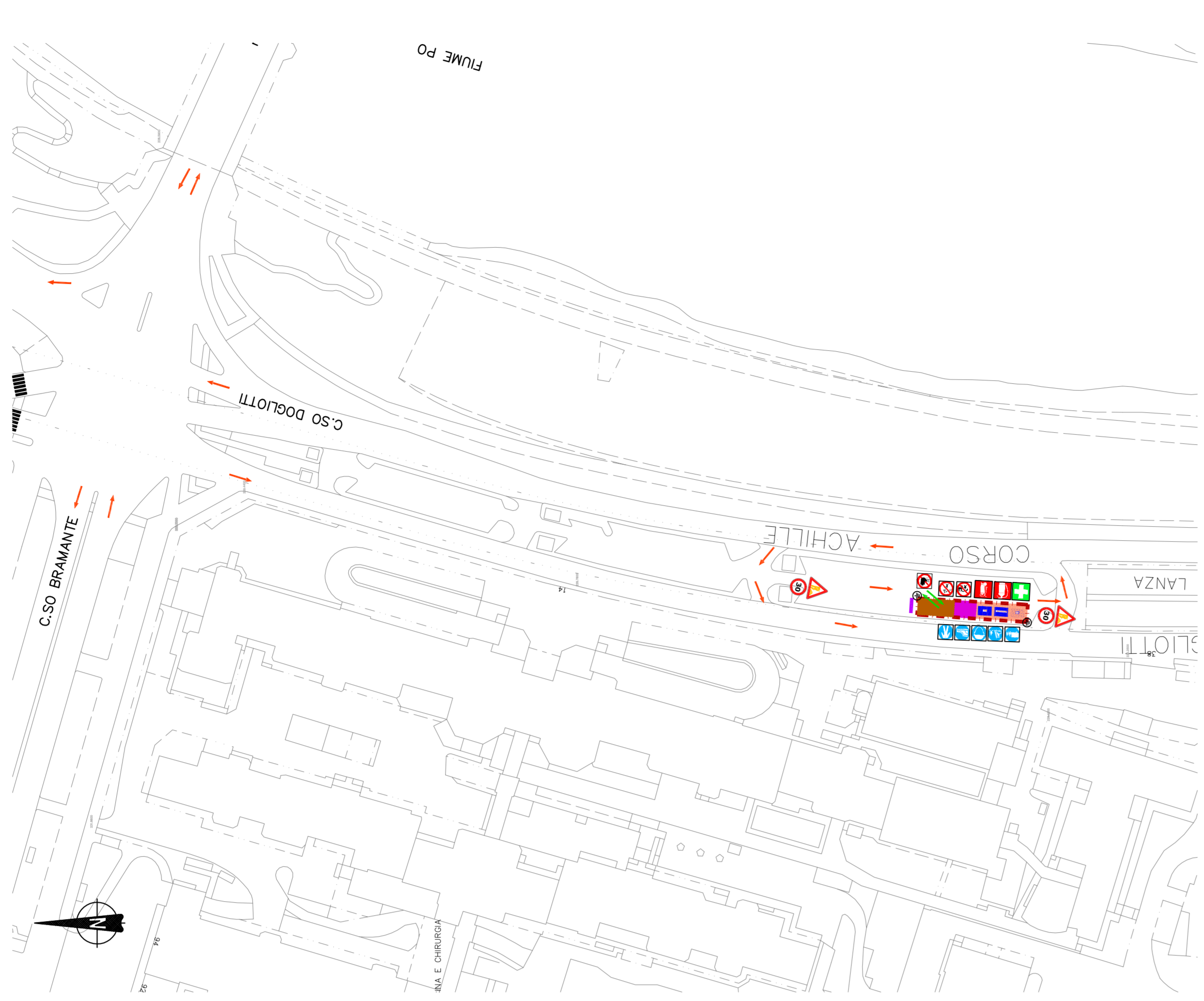
PLANIMETRIA AREA DI CANTIERE - ESTRADOSSO SOTTOPASSO SCALA 1:1000
