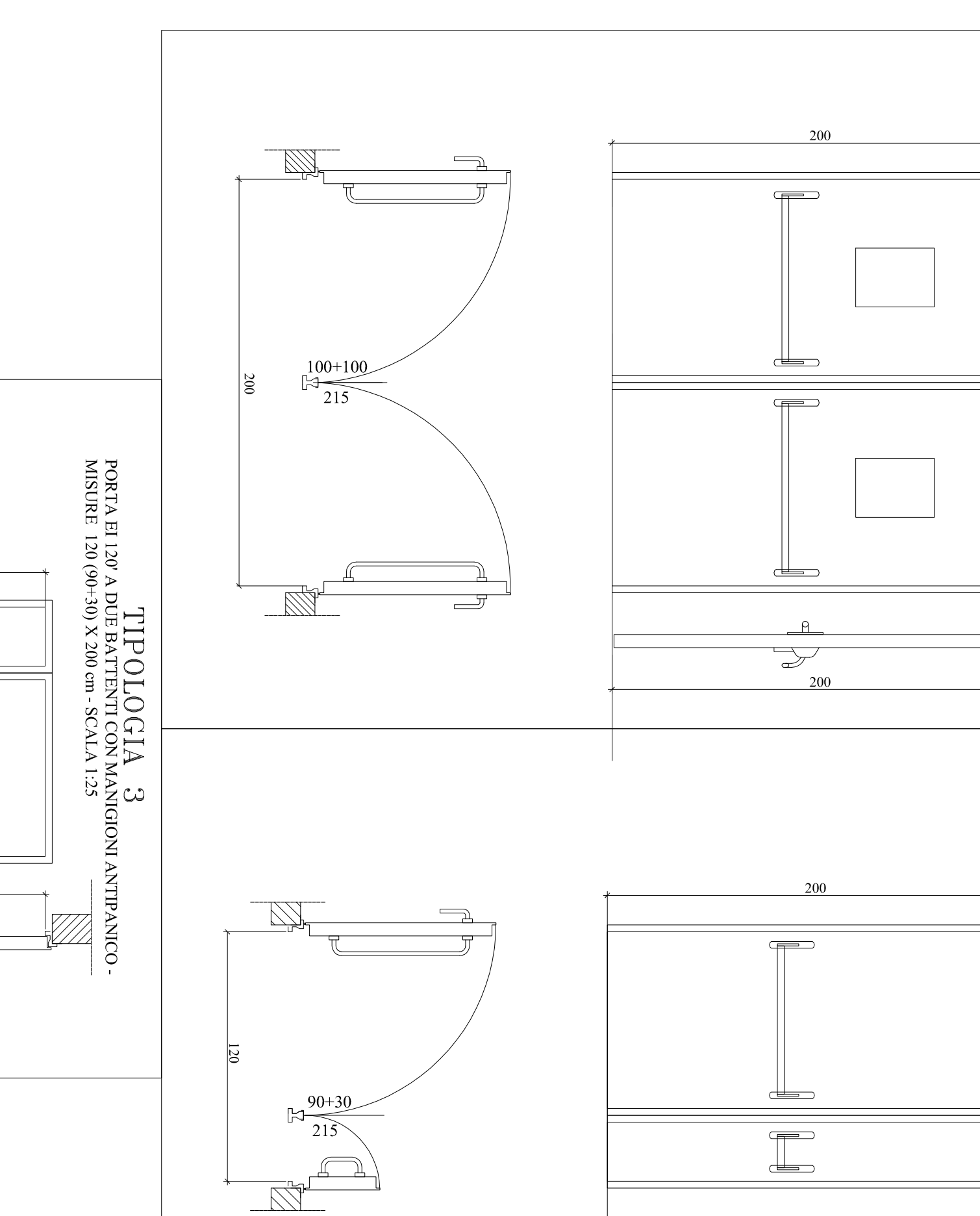
AMCO PORTE TAGLIAFUOCO SCALA 1:25
