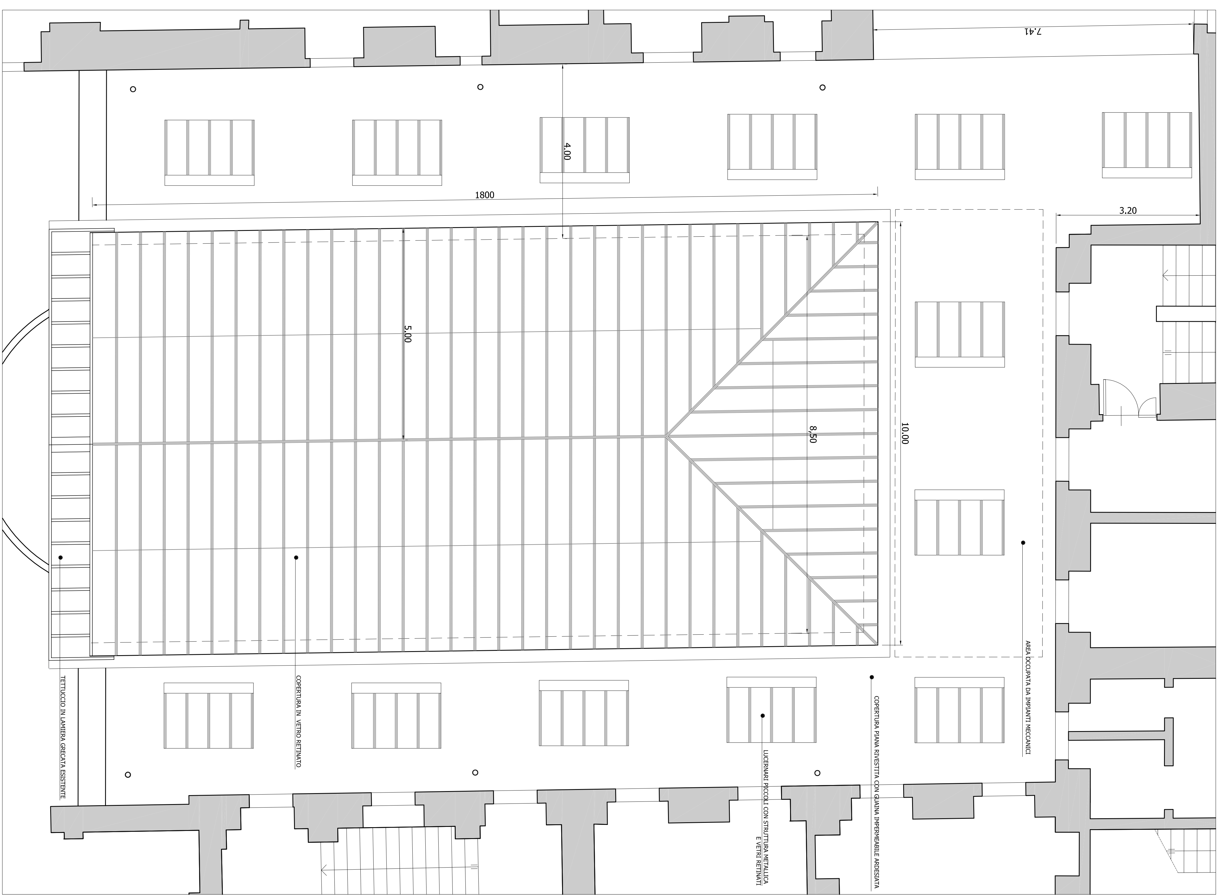
PIANTA STATO ATTUALE COPERTURA "SALA CARPANINI" scala 1:50
