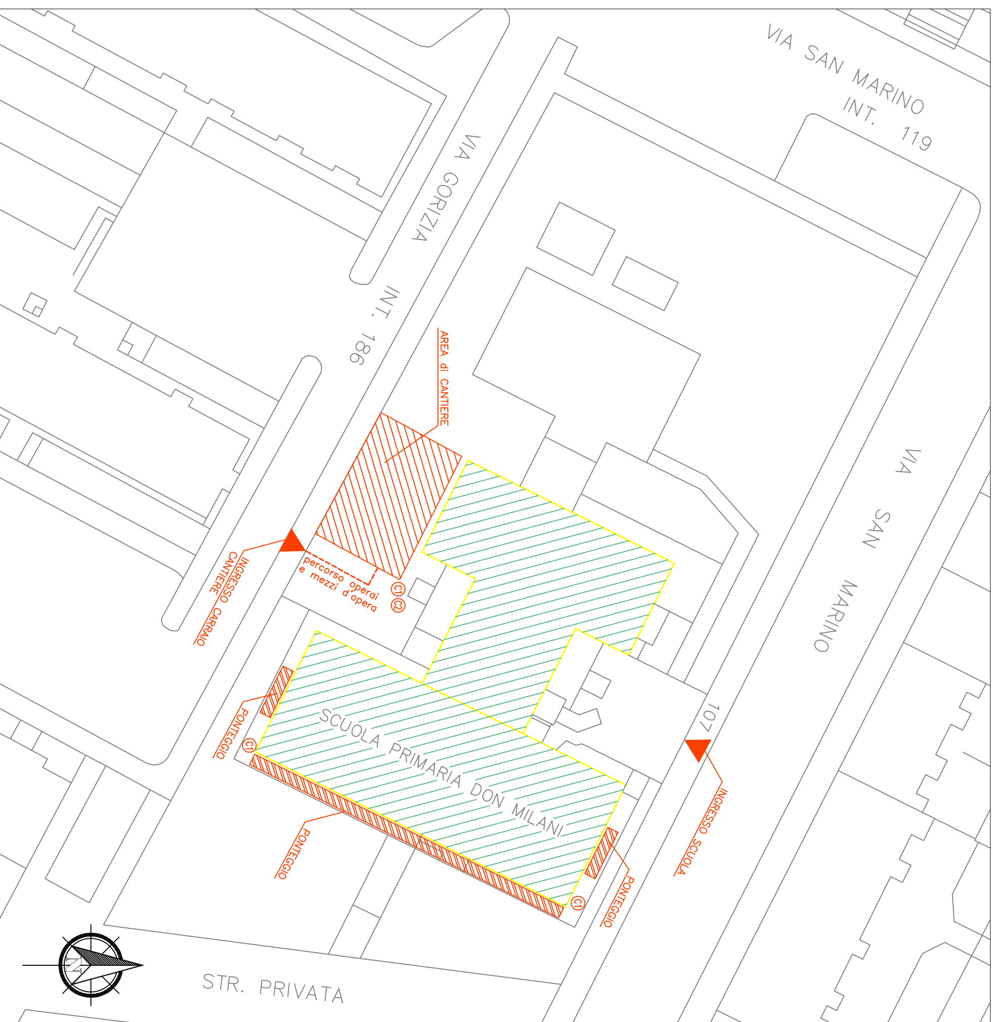
PLANIMETRIA - scala 1:500
