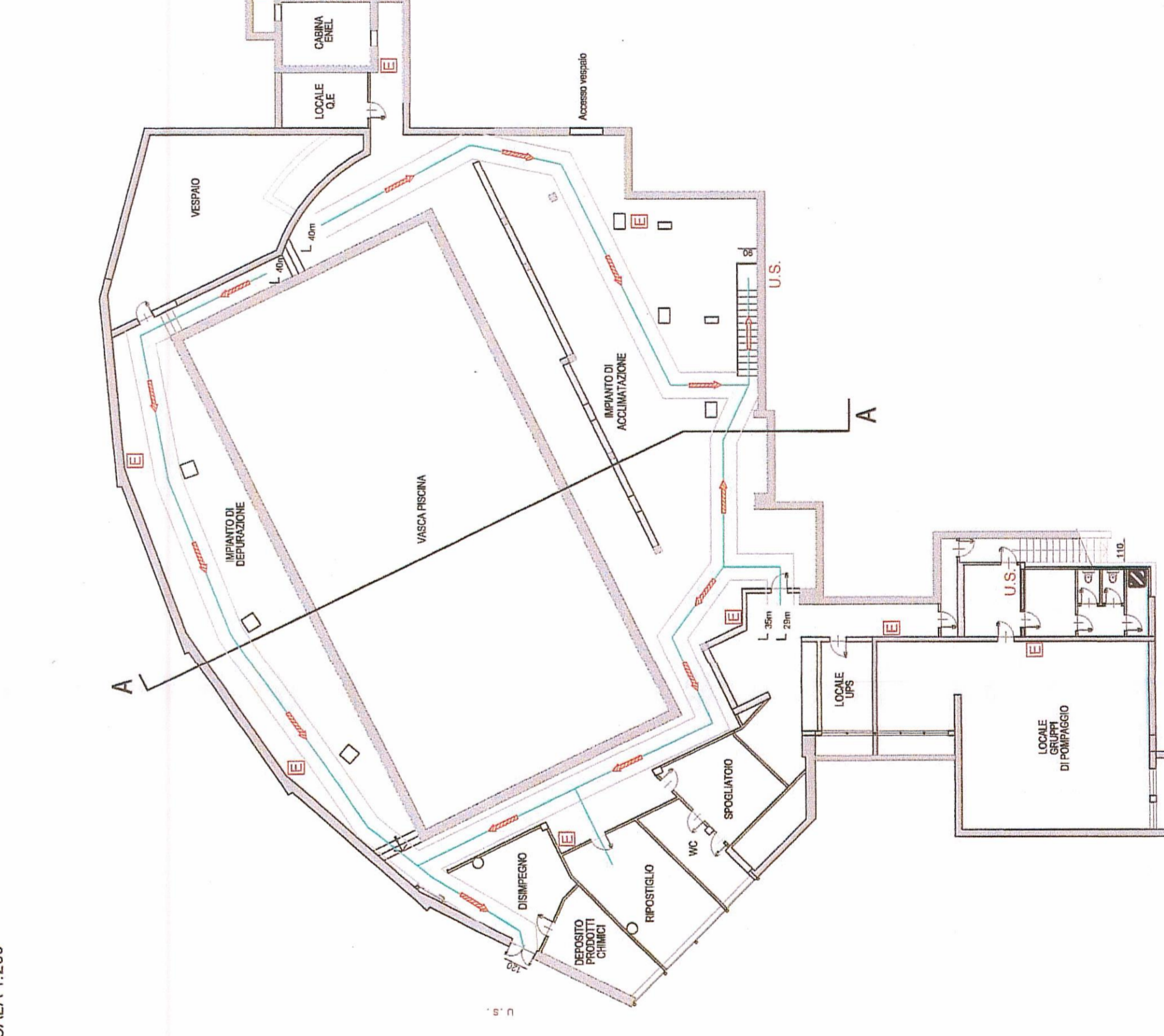
PLANIMETRIA PIANO INTERRATO SCALA 1:200
