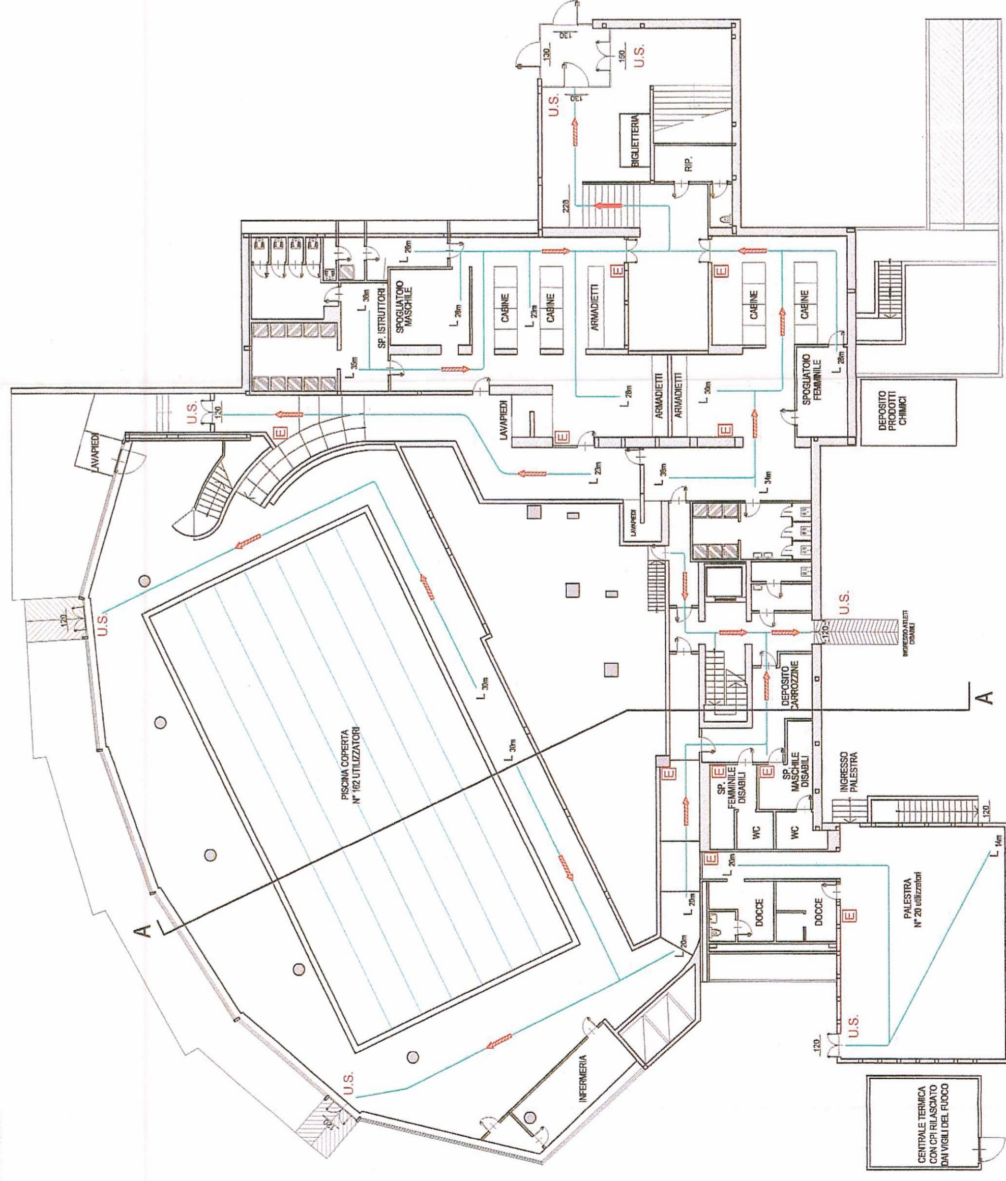
PLANIMETRIA PIANO SEMINTERRATO SCALA 1:200
