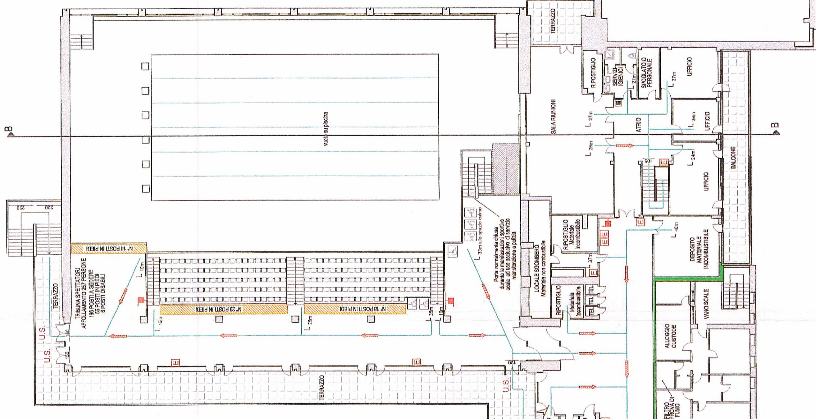
PLANIMETRIA PIANO PRIMO SCALA 1:200
