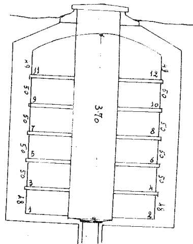
SEZIONE CD
