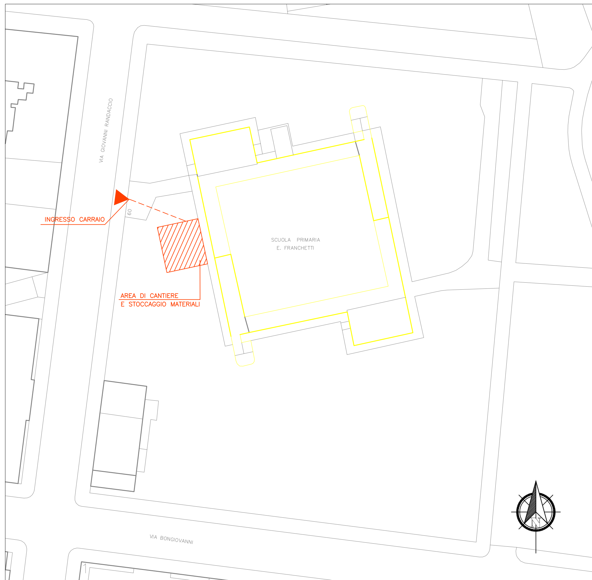
PLANIMETRIA - scala 1:500
