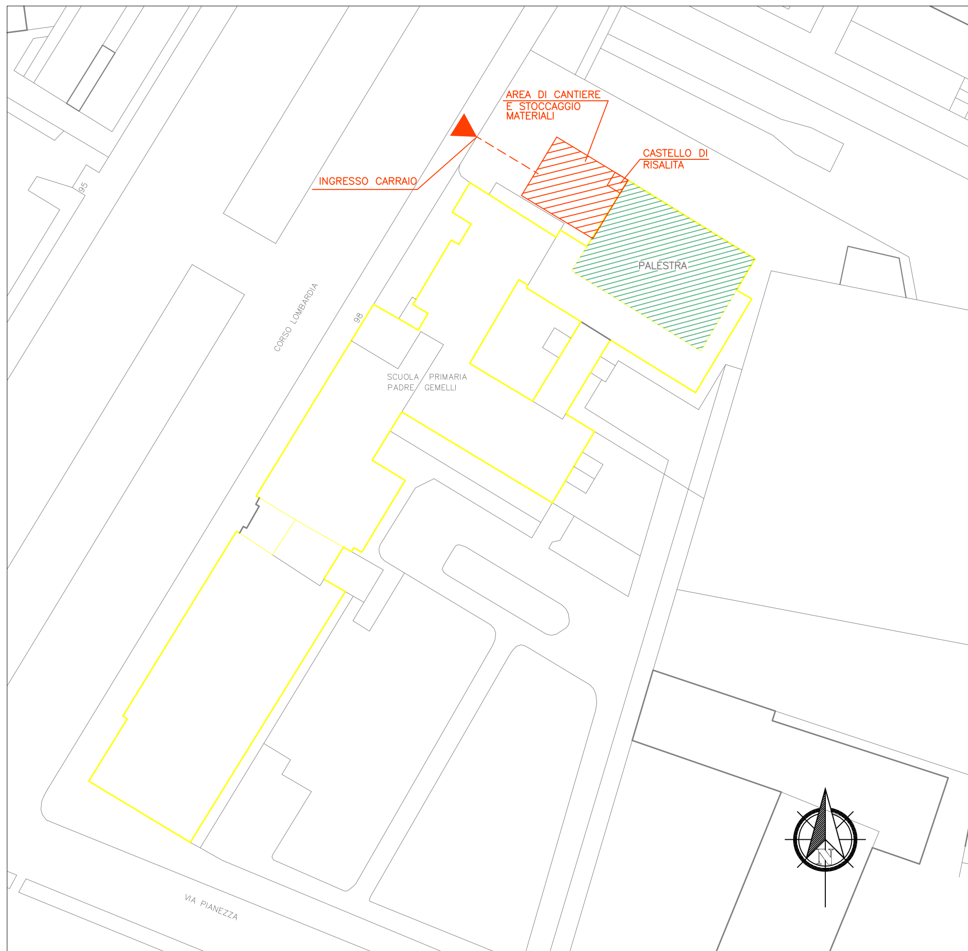
PLANIMETRIA - scala 1:500
