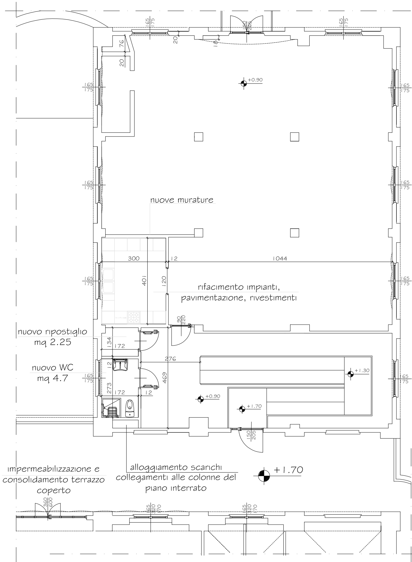
MANUTENZIONE STRAORDINARIA LOCALE "OASI" VIA SAN MARINO 10_PIANTA PROGETTO_SCALA 1:100
