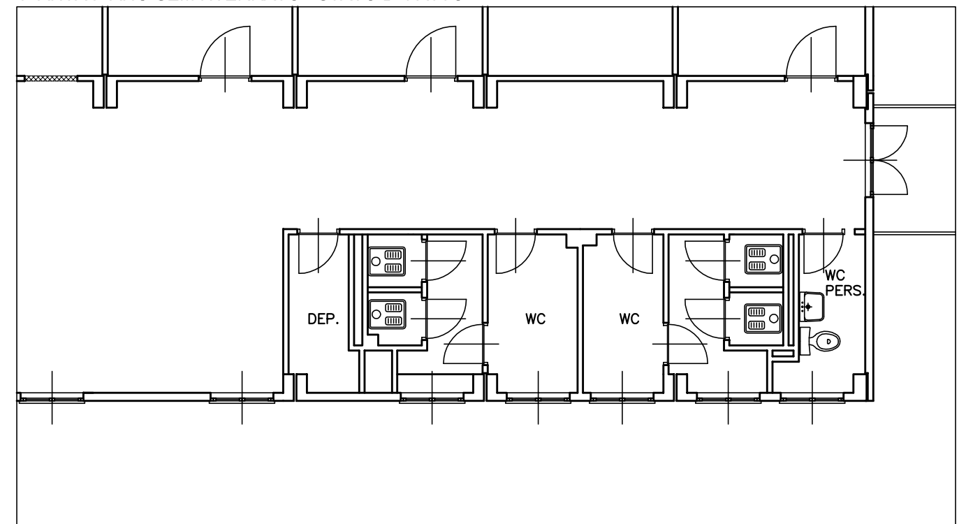
PIANTA PIANO SEMINTERRATO - PROGETTO
