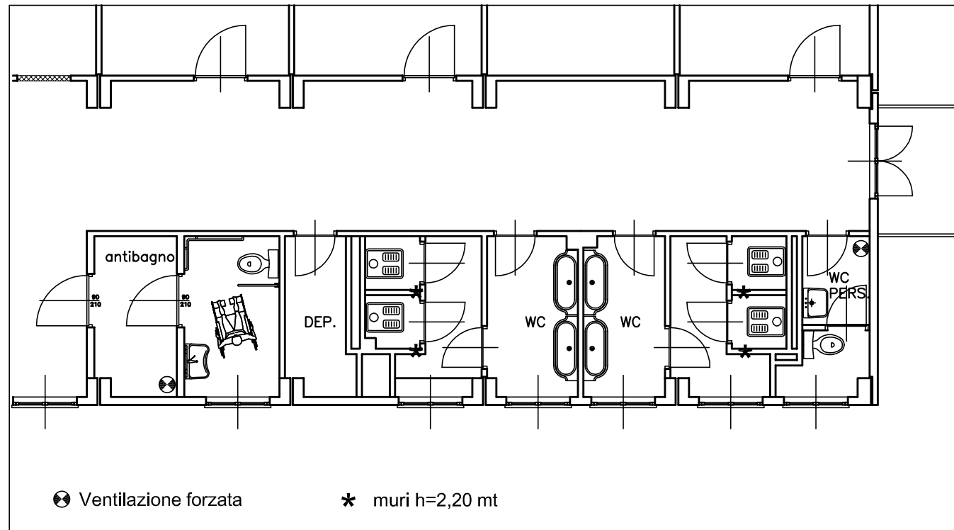
PIANTA PIANO RIALZATO - PROGETTO
