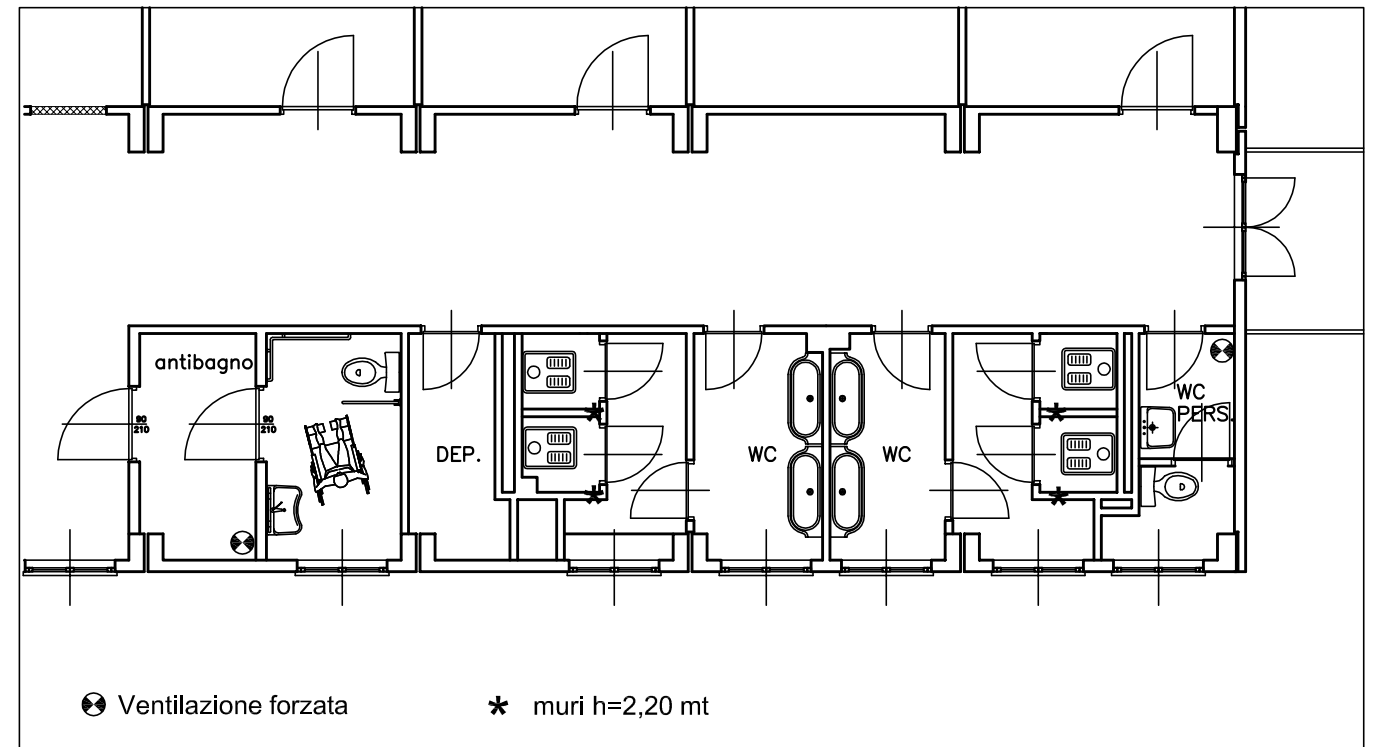
PIANTA PIANO SECONDO - PROGETTO
