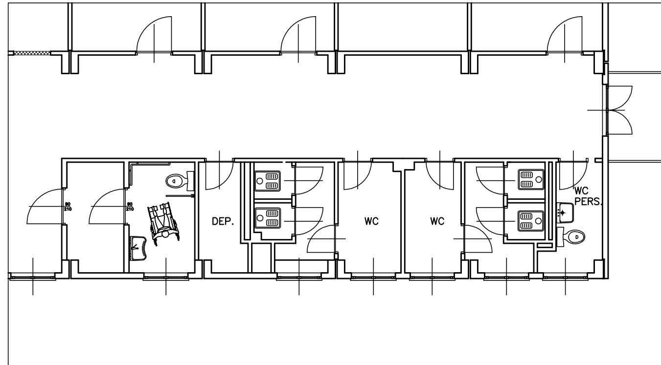
PIANTA PIANO PRIMO - PROGETTO
