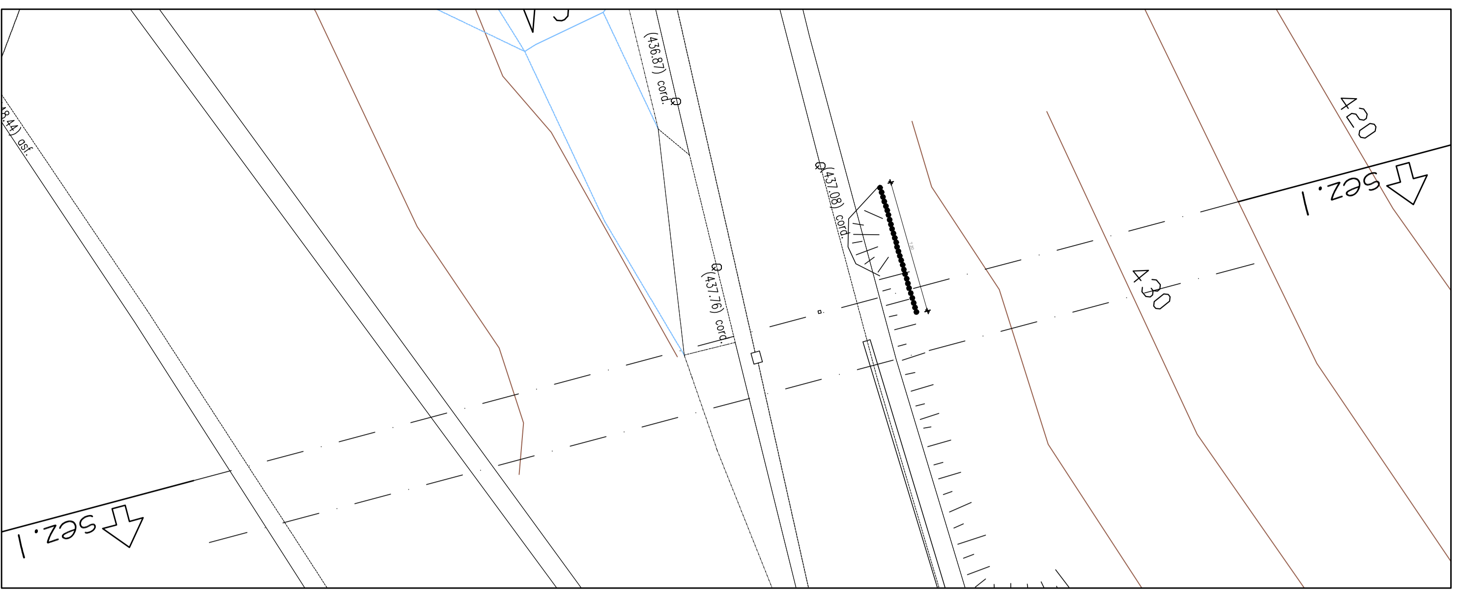
Planimetria scala 1:200
