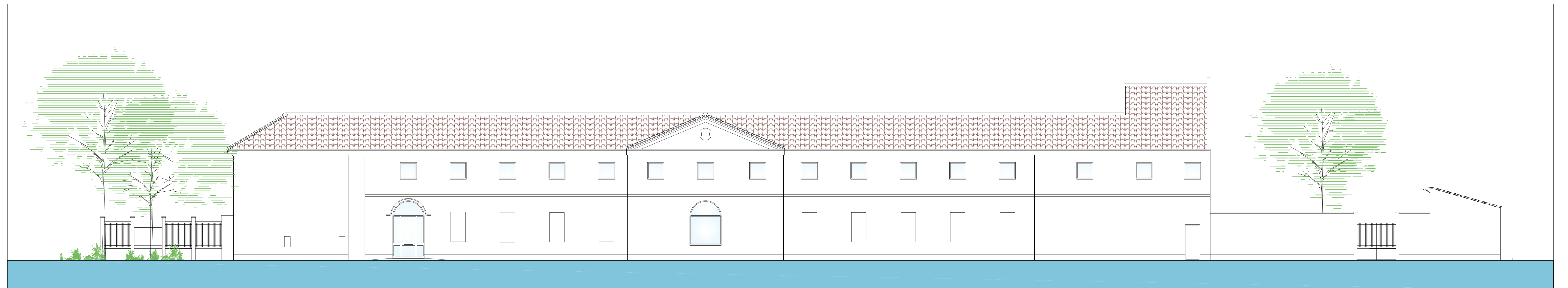
Prospetto manica centrale Via Sambuy
