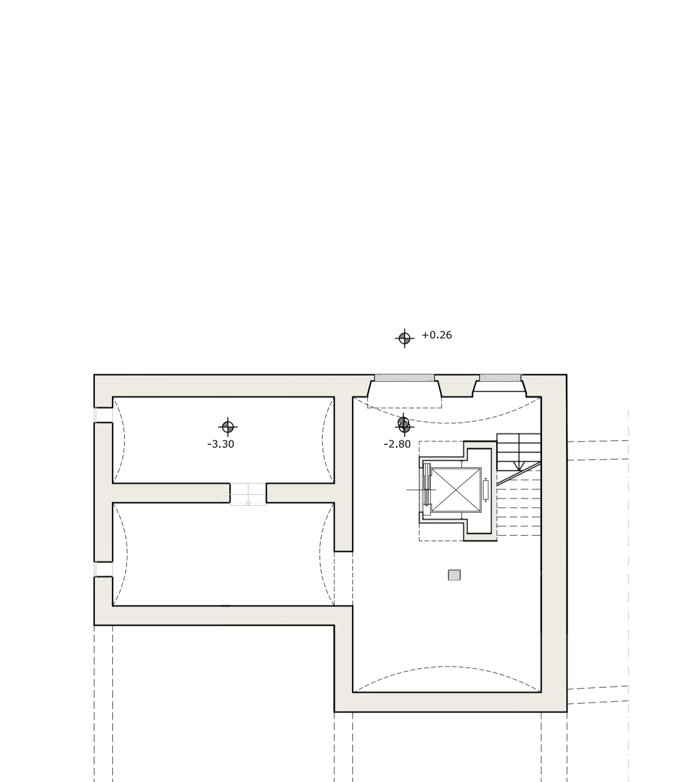
PIANTA PIANO CANTINATO
