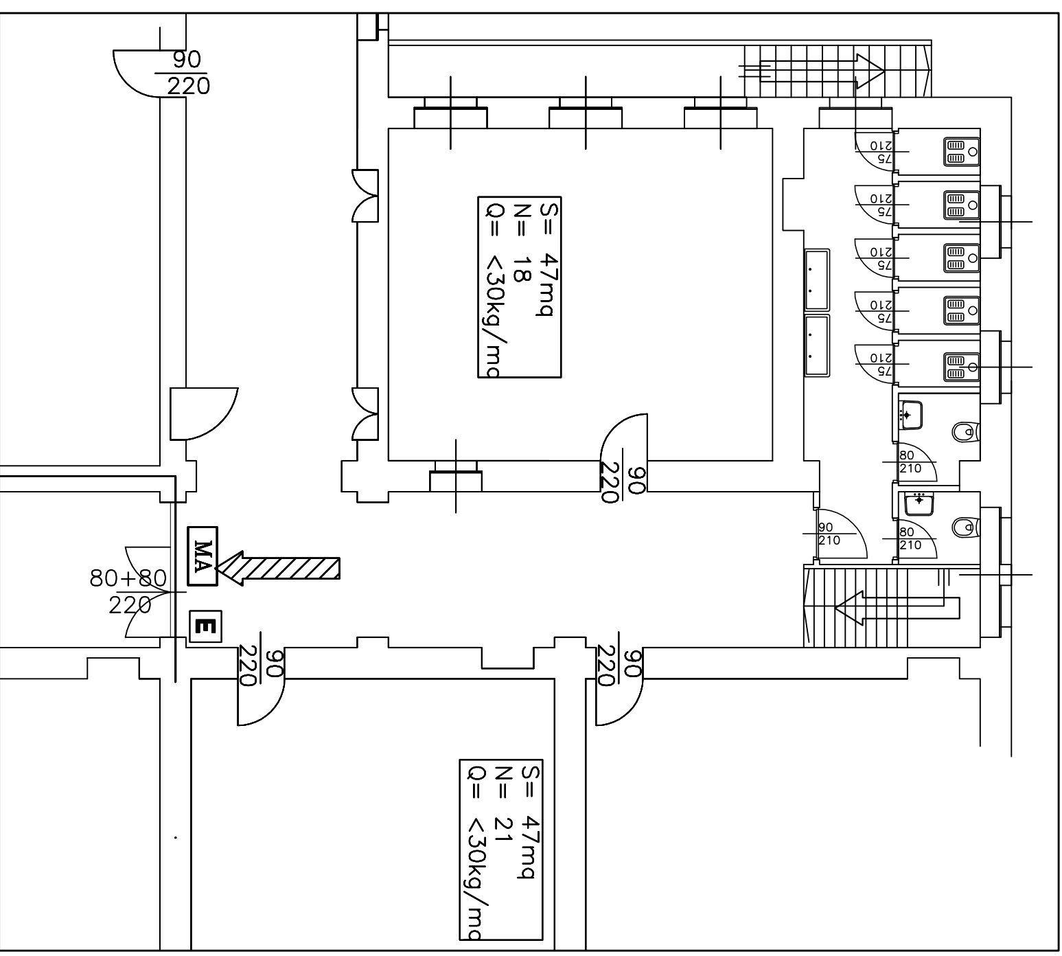
SERVIZI LATO EST PROGETTO
