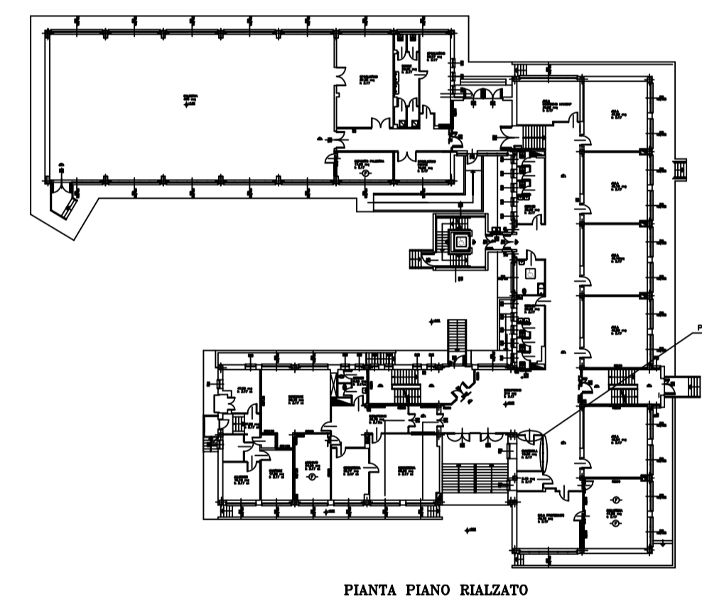
PIANTA PIANO RALZATO
