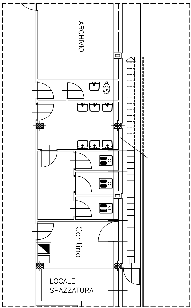
PIANTA PIANO SEMINTERRATO - STATO DI FATTO
