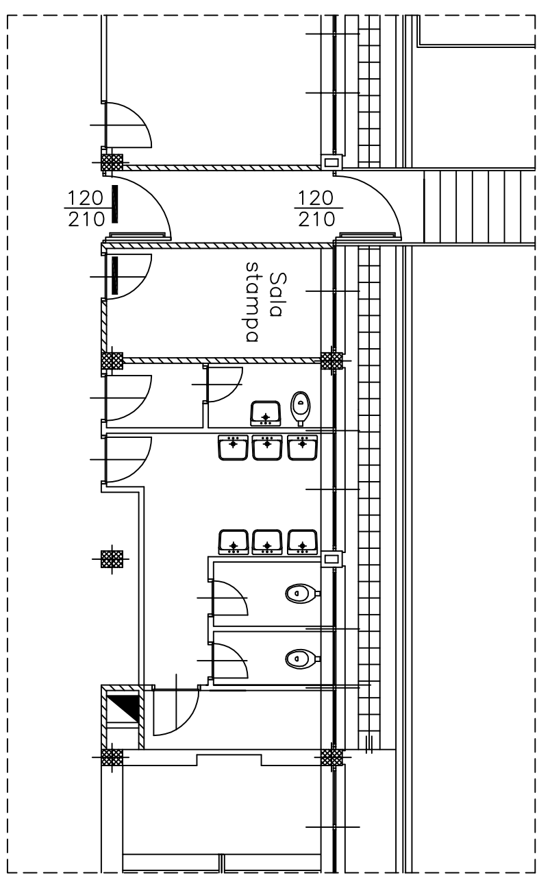
PIANTA PIANO RIALZATO - STATO DI FATTO
