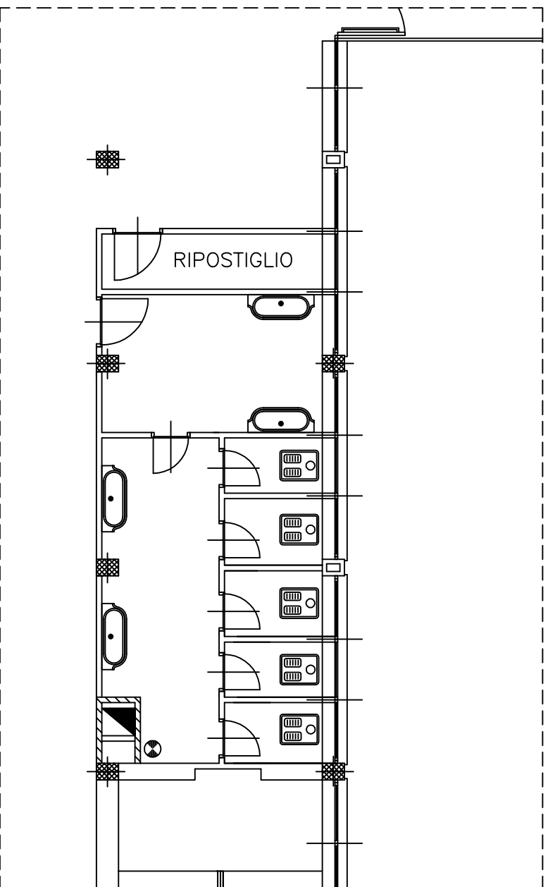
PIANTA PRIMO PIANO - PROGETTO
