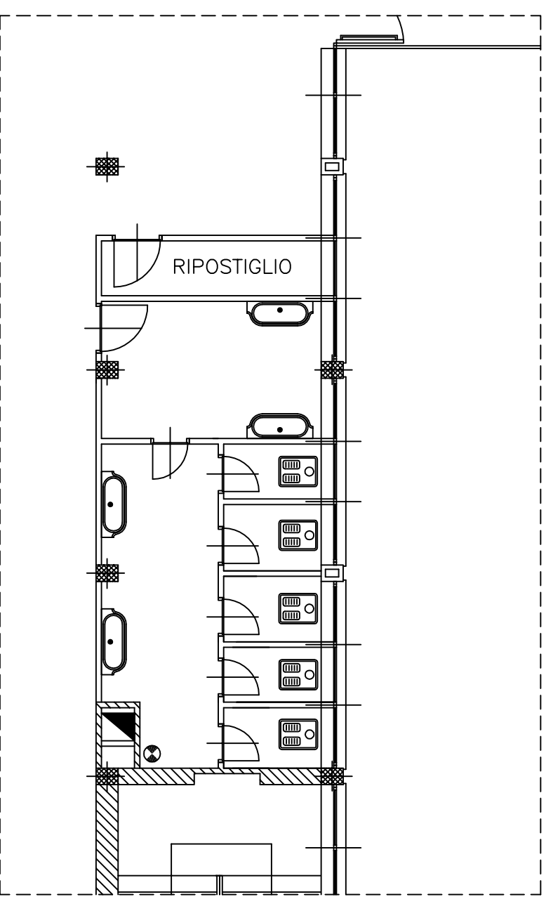
PIANTA SECONDO PIANO - PROGETTO
